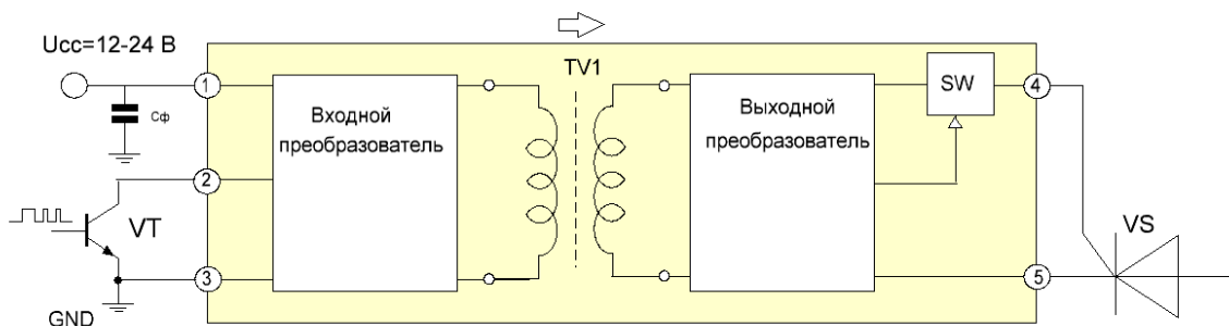
Рисунок 2. Функциональная схема
