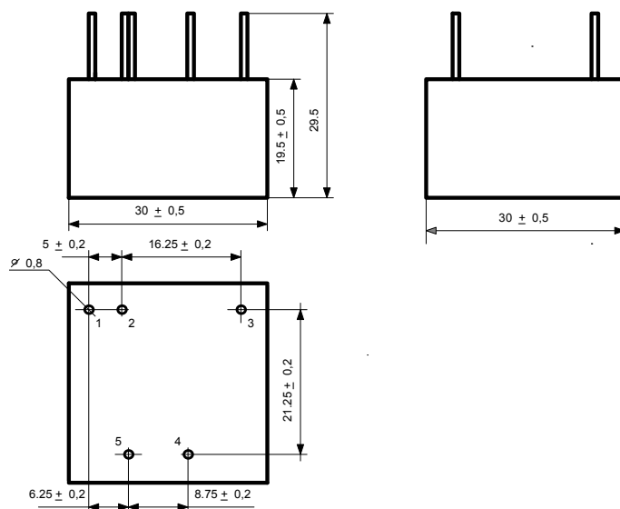
Рисунок 1. Габаритный чертёж
